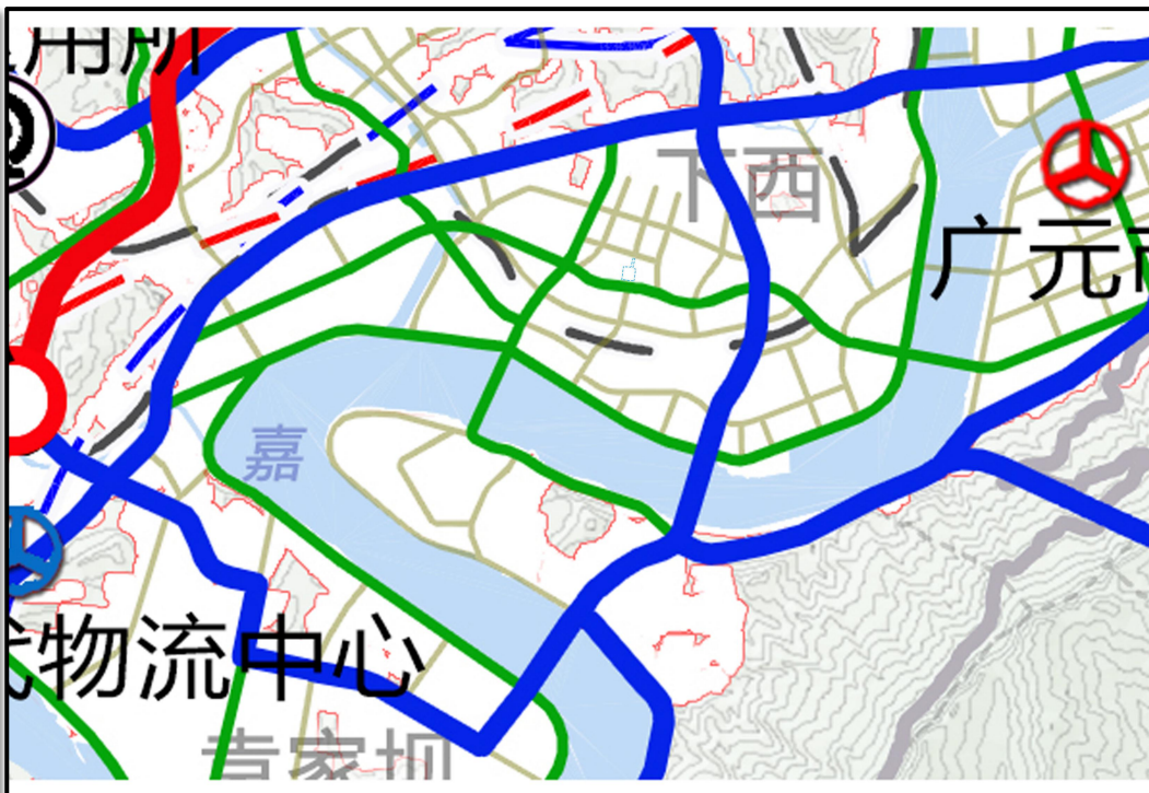
38中心城区道路交通规划图
